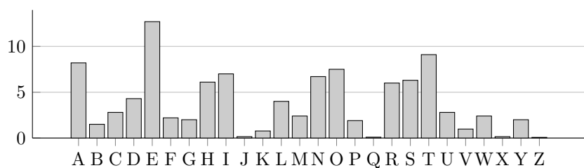
Četnost písmen v anglickém jazyce v %
