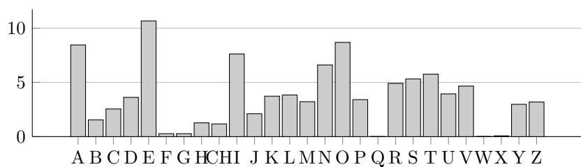
Četnost písmen v českém jazyce v % 1
